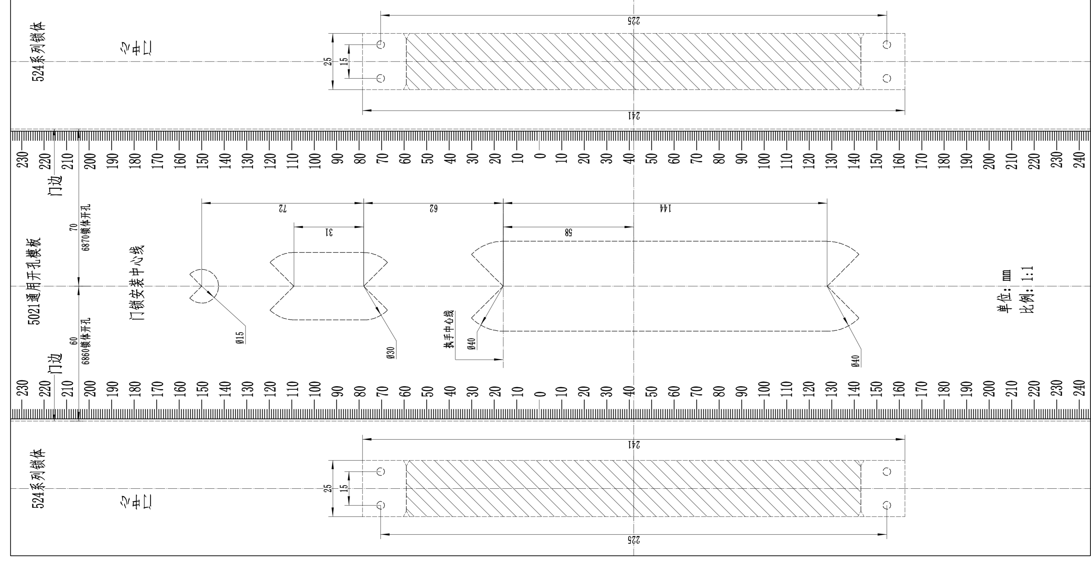
正面图
